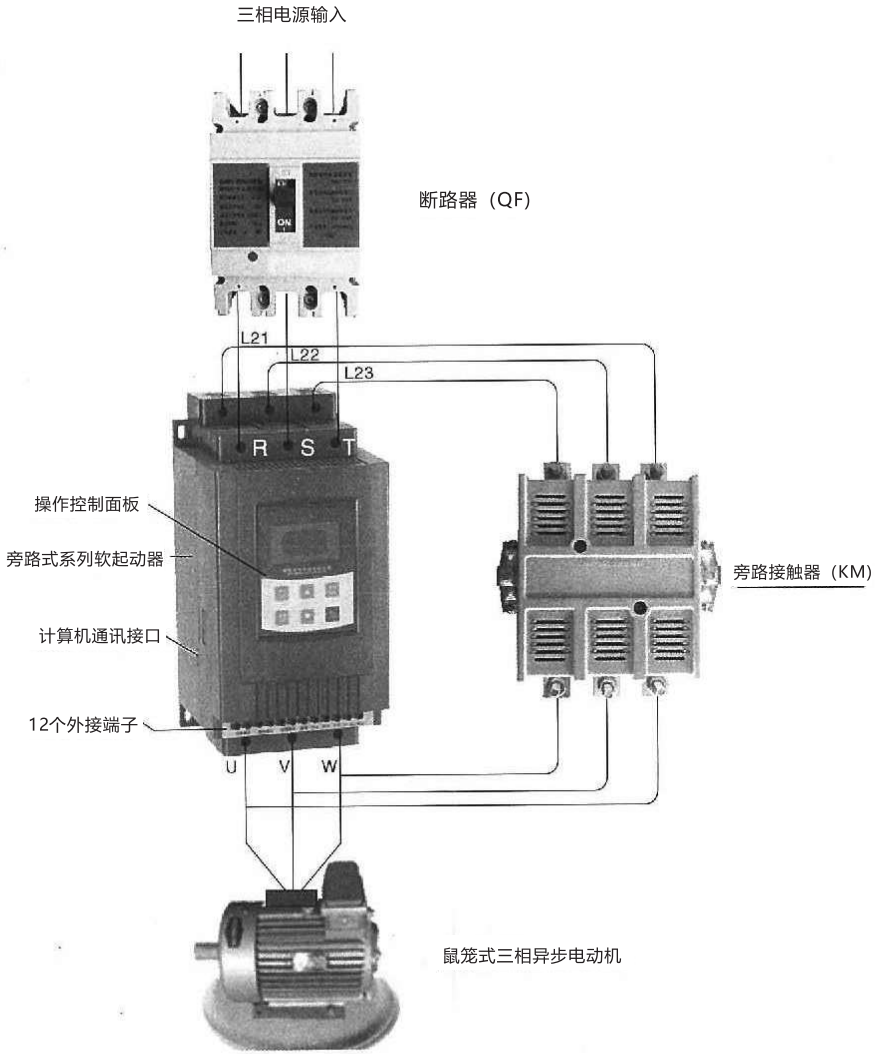
基本接线示意图
